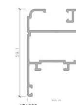
451003 HOJA PARA VENTANA BATIENTE Y PROYECTANTE INTERIOR Y EXTERIOR.
