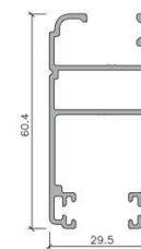
452002 HOJA PARA CORREDERA.
