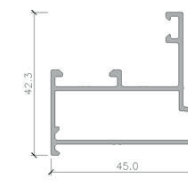
451001 MARCO PARA BATIENTE Y PARO FIJO 45 MM.
