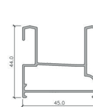
452001 MARCO PARA CORREDERA 45 MM.
