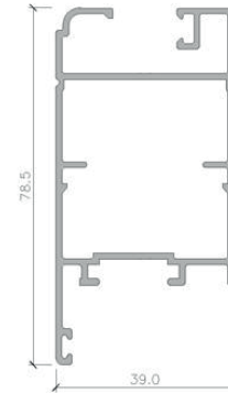
451002 HOJA PARA PUERTA BATIENTE INTERIOR Y EXTERIOR.
